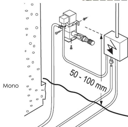
Clapet d'air avec électrovanne
