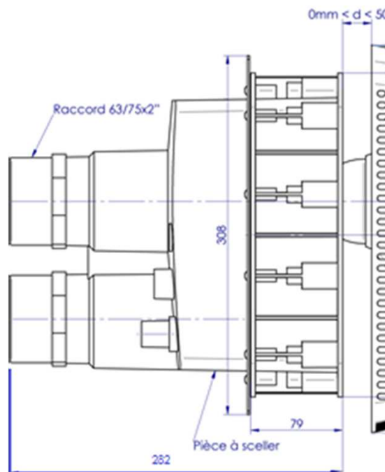
Clapet d'air avec électrovanne
